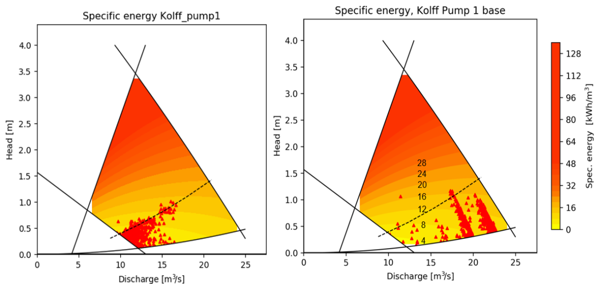
FIGUUR 6.4 POMPWERKPUNTEN EN SPECIFIEKE ENERGIE (KWH/M 3 ) VOOR POMP 1 VAN KOLFGEMAAL IN 2013 VOOR HET GEOPTIMALISEERDE MODEL (LINKS) EN HET REFERENTIE-MODEL (RECHTS). DE BEGRENZING VAN HET WERKGEBIED WORDT BEPAALD DOOR HET MINIMALE EN MAXIMALE POMPTOERENTAL EN EEN MINIMAAL RENDEMENT VAN 50%. DE STIPPELIJN TOONT DE WERKPUNTEN MET HET HOOGSTE POMPRENDEMENT
