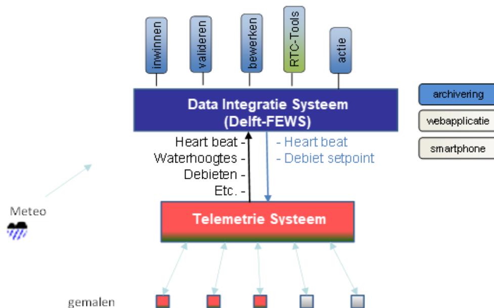
FIGUUR 8.1 SYSTEEMOVERZICHT SLIM MALEN
