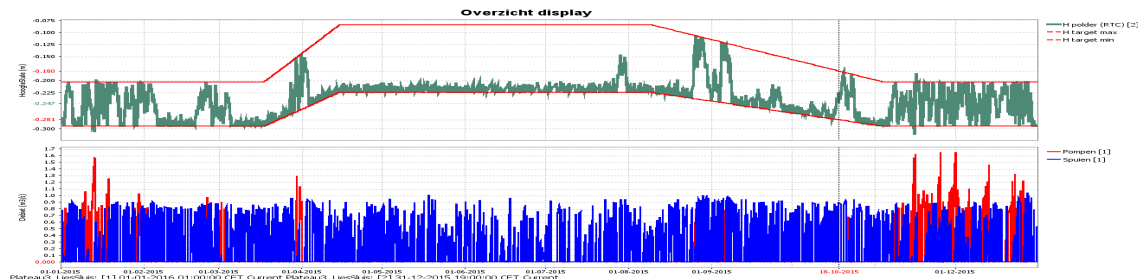
FIGUUR 6.3 INZET VAN POMPEN (ROOD) EN SLUIZEN (BLAUW) BIJ LIESSLUIS IN HET JAAR 2015
