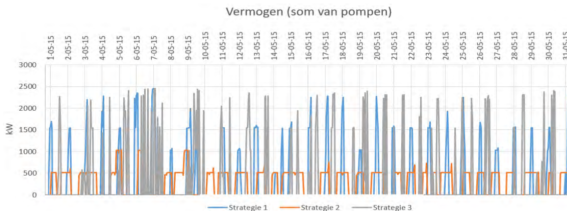
FIGUUR 6.2 INZET VAN POMPEN IN DE VERSCHILLENDE SCENARIO'S OVER DE MAAND MEI. STRATEGIE 1 OPTIMALISEERT ENERGIEKOSTEN, STRATEGIE 2 HET ENERGIEVERBRUIK EN STRATEGIE 3 OPTIMALISEERT OOK OP ENERGIEKOSTEN, MAAR GEEFT VOORRANG AAN DE LOKALE OPWEK VAN EEN WINDMOLEN
