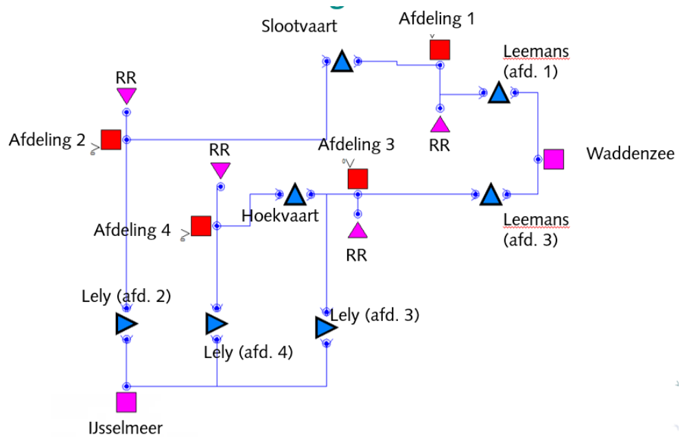
FIGUUR 6.1 SCHEMATISATIE VAN DE WIERINGERMEERPOLDER IN RTC-TOOLS
