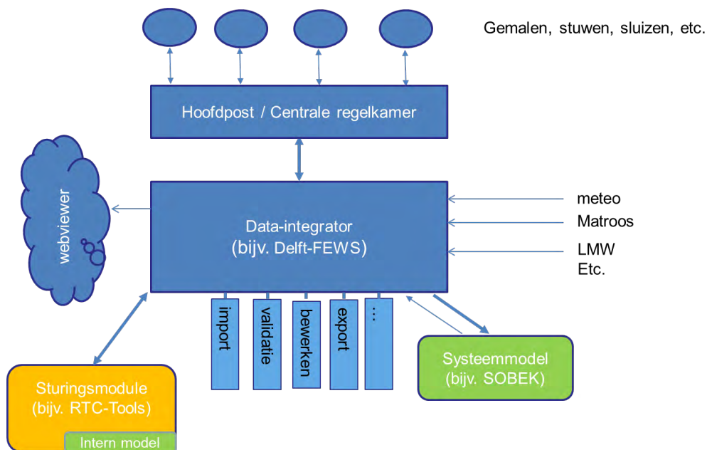
ELEMENTEN IN EEN OPERATIONEEL WATERBEHEERSYSTEEM
